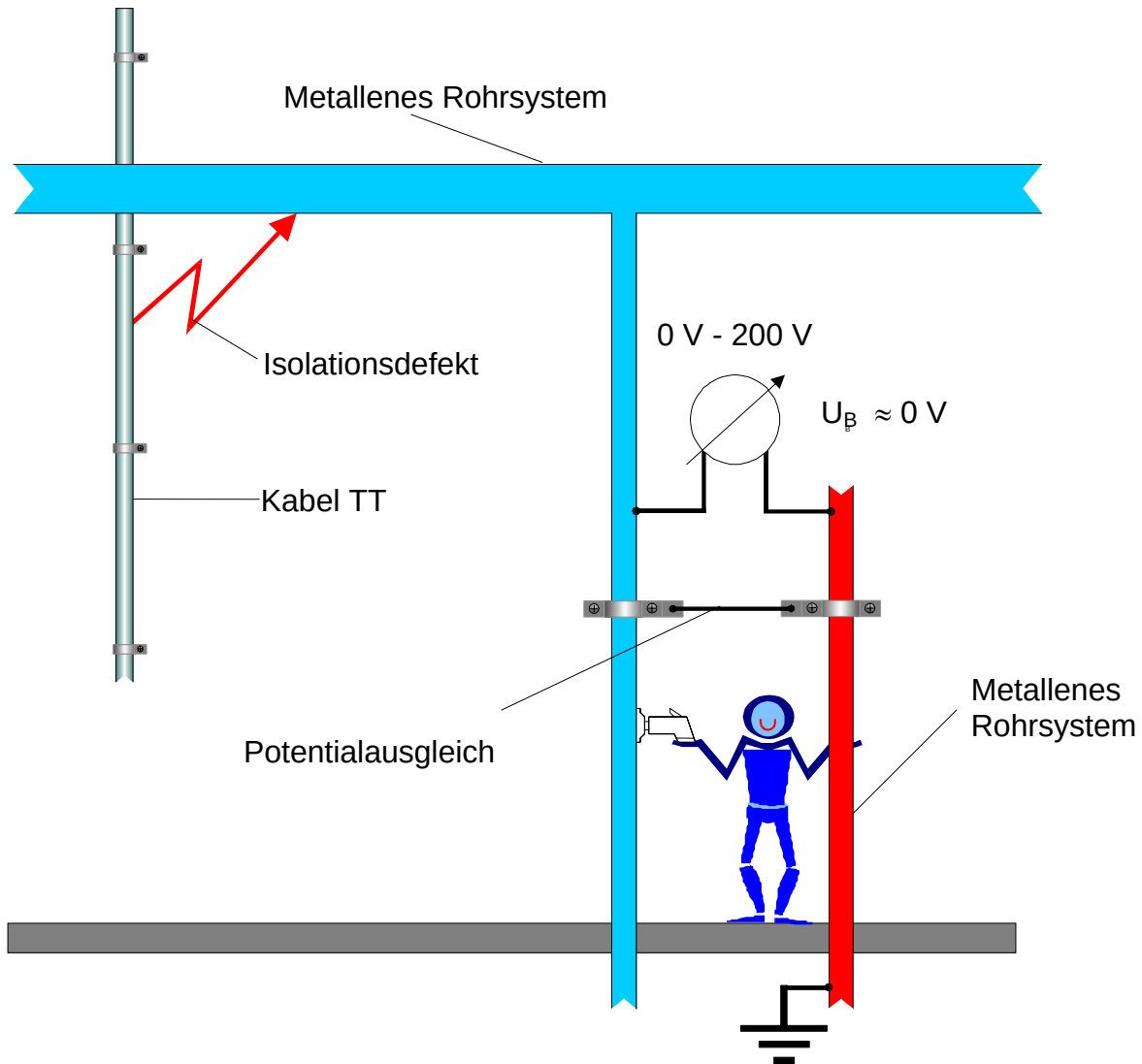
Abb. 1.2 Anlage mit Potentialausgleich
