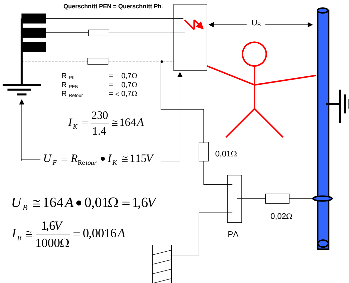
Abb. 2.2.1 Berührungsspannung mit Potentialausgleich
