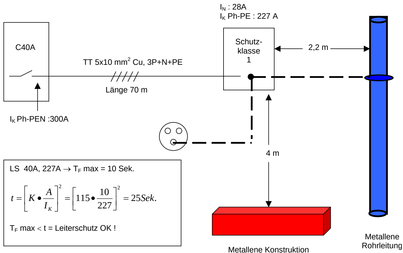
Abb. 5.1 Zusätzliche Potentialausgleiche
