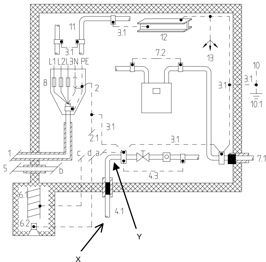
Abb. 3.1 Beispiel aus NIN 1000-2, Art. 41411
