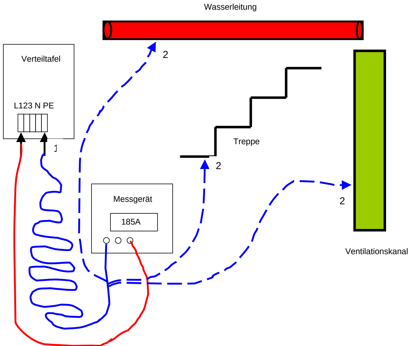
Abb. 6.1 Kontrolle des Potentialausgleichs
